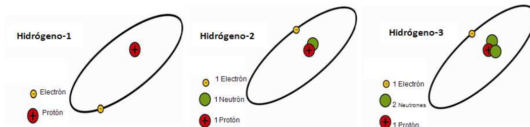
Figura 2.- Isótopos de Hidrógeno
