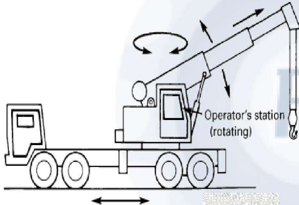
GRÚA SOBRE RUEDAS Pluma Telescópica
