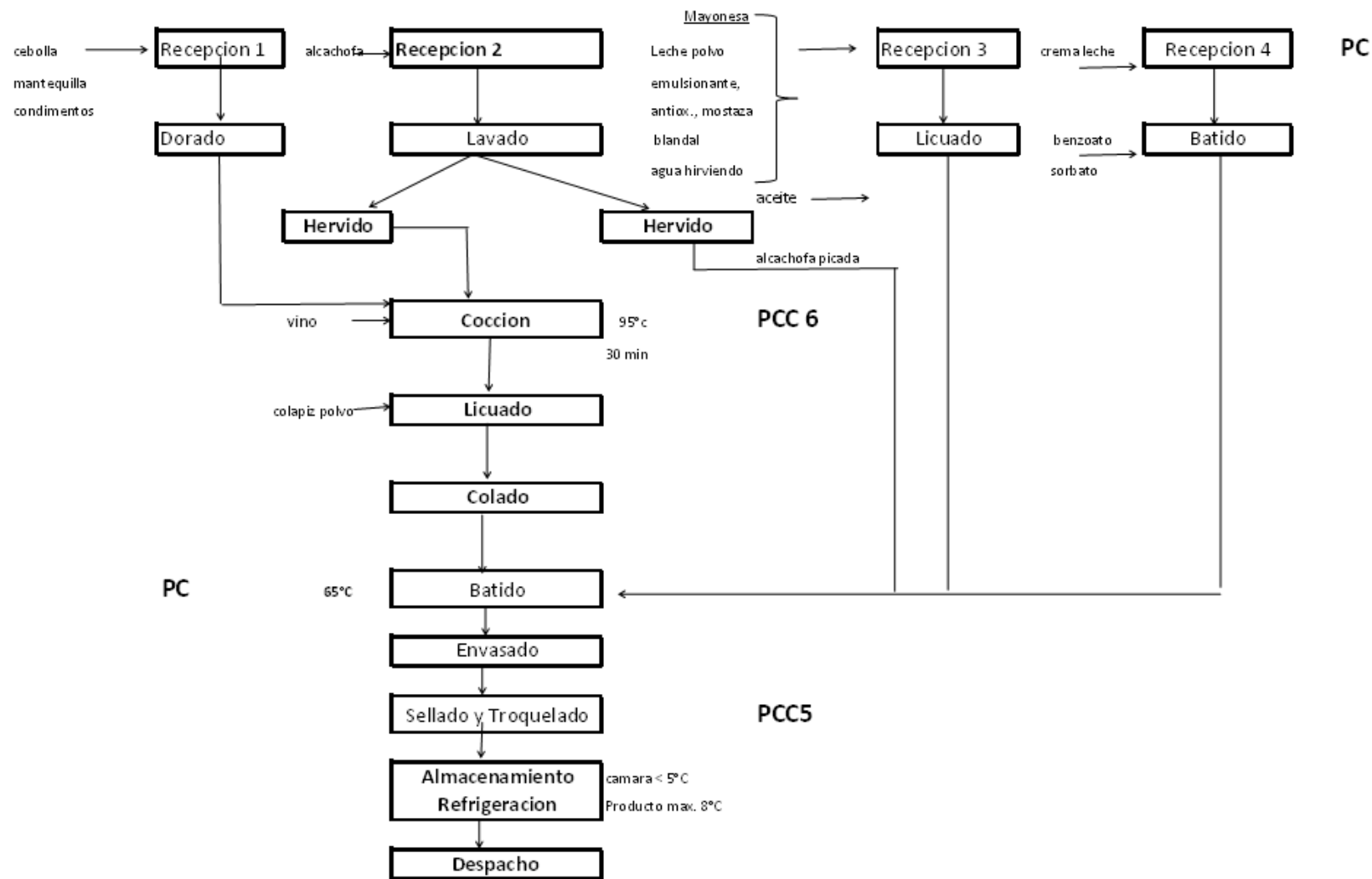
DIAGRAMA 4: FLUJO PROCESO PATE ALCACHOFA
