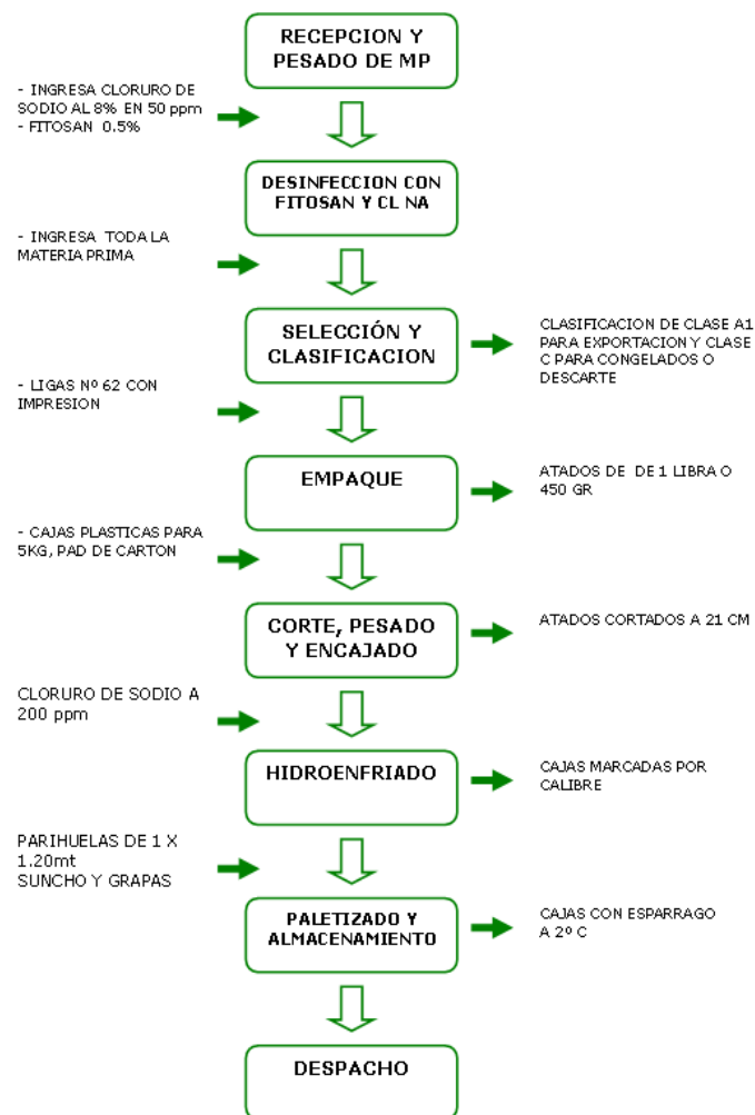
DIAGRAMA DE FLUJO DE PRODUCCION DEL ESPARRAGO VERDE FRESCO DE EXPORTACION
